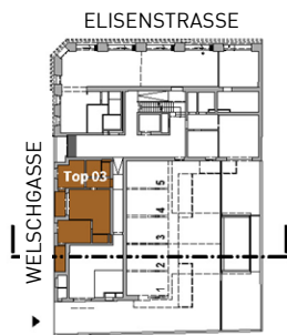
GRUNDRISS (EG)
