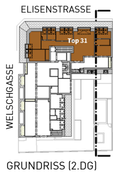
GRUNDRISS (2.DG)
